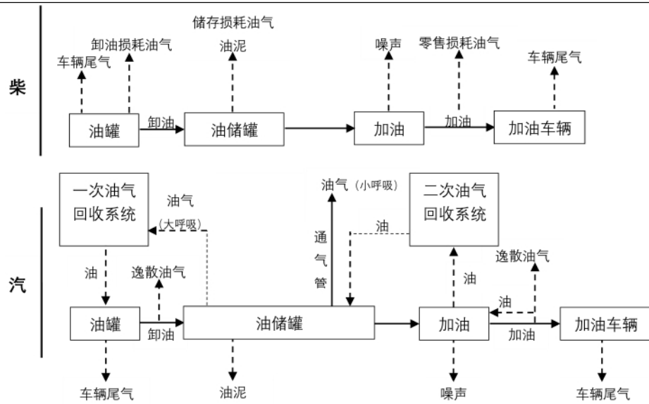
图 5-2 运营期工艺流程及产污节点图
