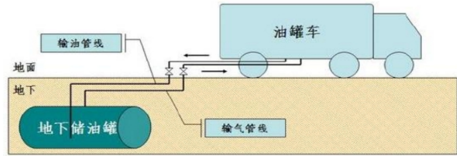
图 5-3 卸油油气回收系统工艺流程图
