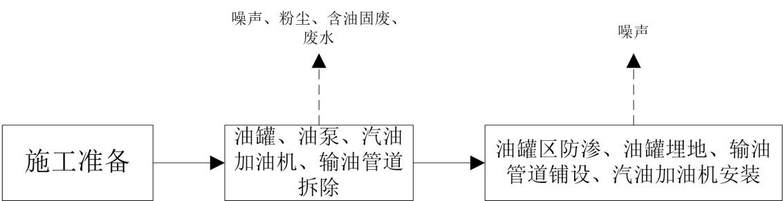
图 5-1 施工期流程及产污环节图
