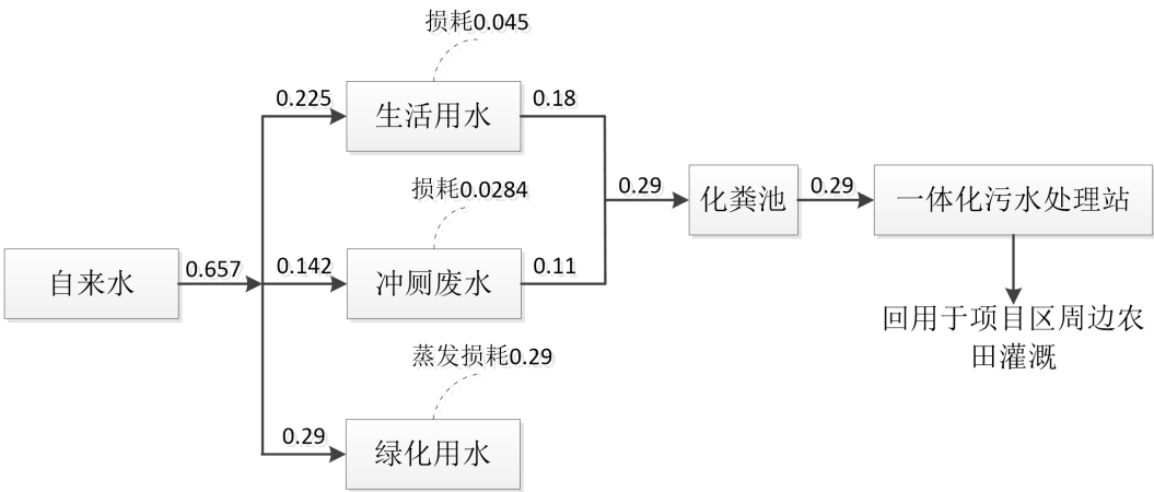
图 5-5 项目晴天水量平衡图 (m³/d)
